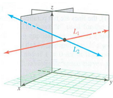
Các đường thẳng cắt nhau
