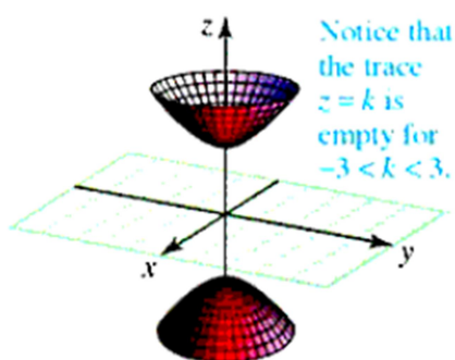
Hình 9.70 Đồ thị của mặt hyperbol 2 nhánh
