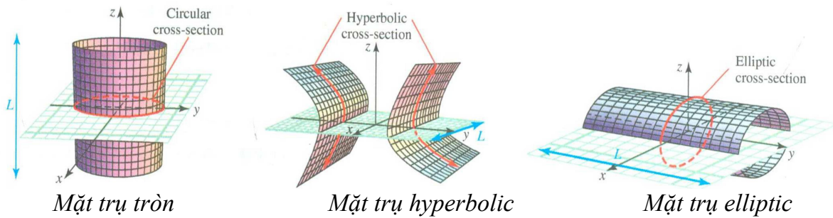
Hình 9.18. Các loại mặt trụ
