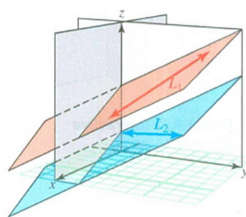
Các đường thẳng chéo nhau
